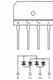
FMS-3FU
