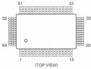
CXA2000Q-TL
