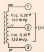
BV 9281-099 Saugkreisspule Absorption Coil Bobine d'absorption
